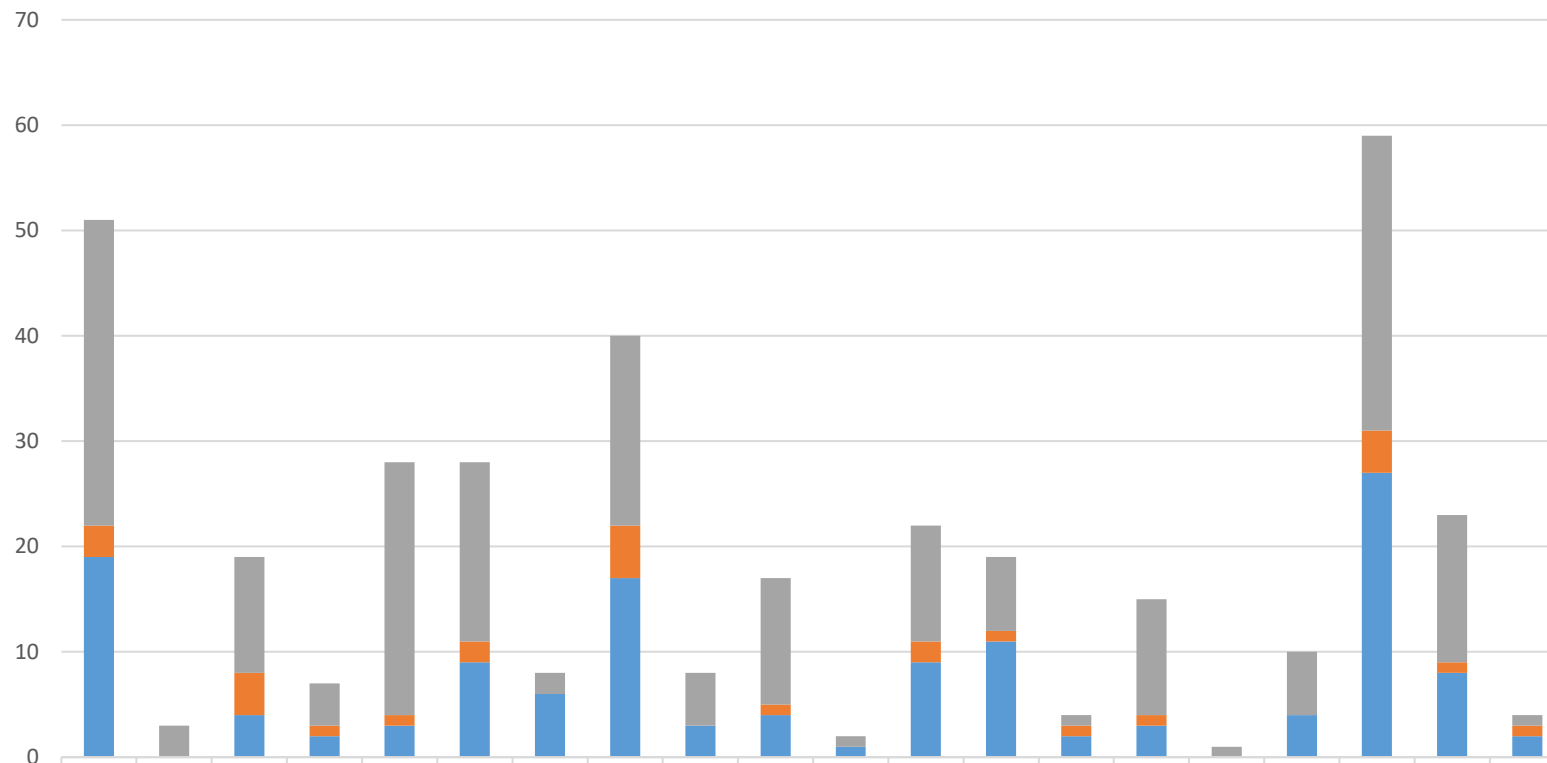
Ergebnisse der vorgezogenen PRIMO-Testung (exls: vorherige Abmeldungen durch Erziehungsberechtigte und Kinder mit Kita-Platz; Stand: 31.01.2022; n=368)
