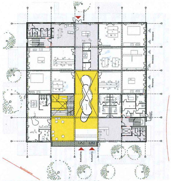
GRUNDRISS ERDGESCHOSS
