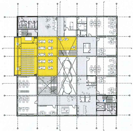
GRUNDRISS 1.OG
