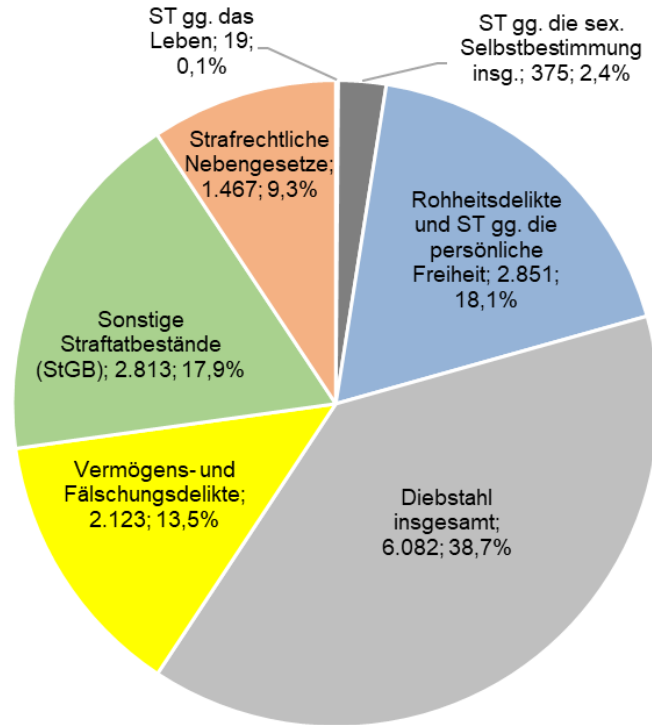
PKS 2024
