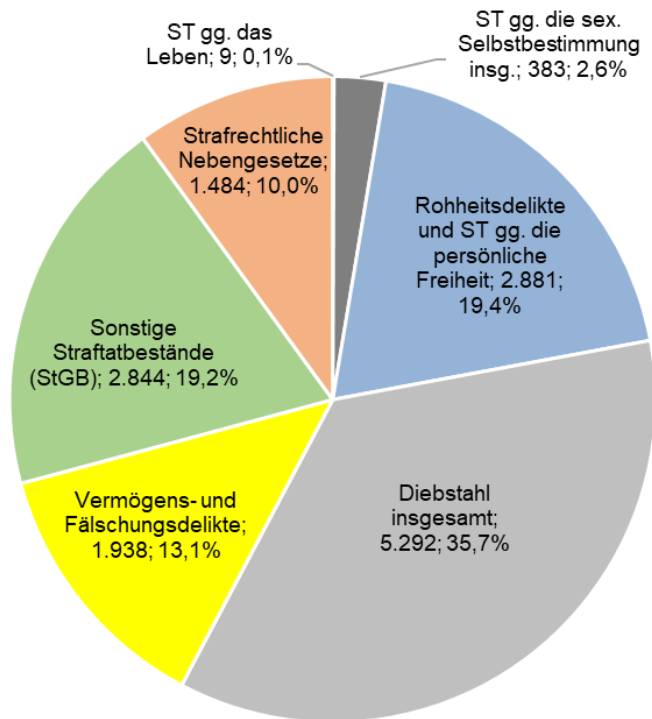
PKS 2023
