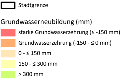
Abb. 43 Belastungskarte Grundwasserneubildung in Bremerhaven
