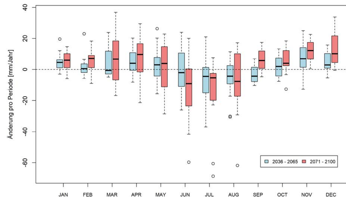
Abb. 25 Änderung der zukünftigen mittleren monatlichen klimatischen Wasserbilanz (Niederschlag minus potenzielle Verdunstung) in Bremen - die Entwicklung in Bremerhaven ist sehr ähnlich (siehe Anhang III)
