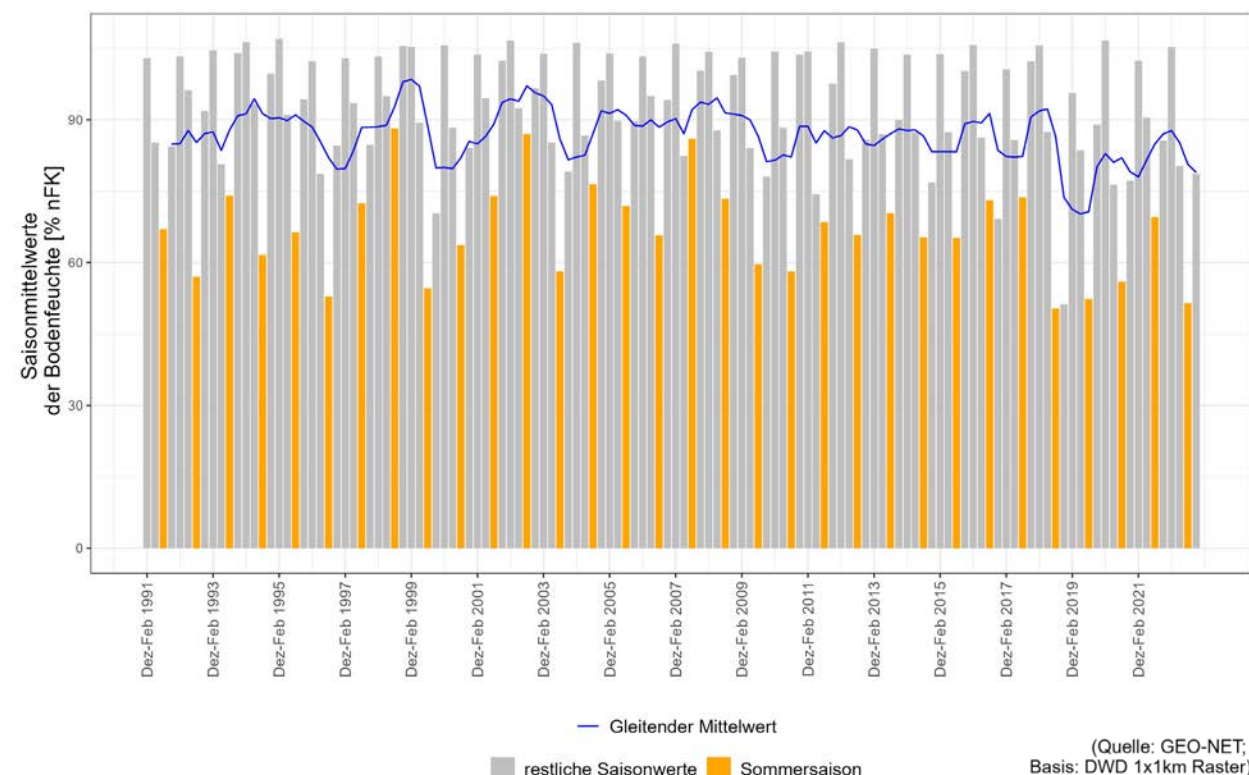
Abb. 24 Entwicklung der saisonalen Mittelwerte der Bodenfeuchte in Bremerhaven im Zeitraum von 1991 bis 2021 – die Entwicklung in Bremen ist sehr ähnlich (siehe Anhang III)
