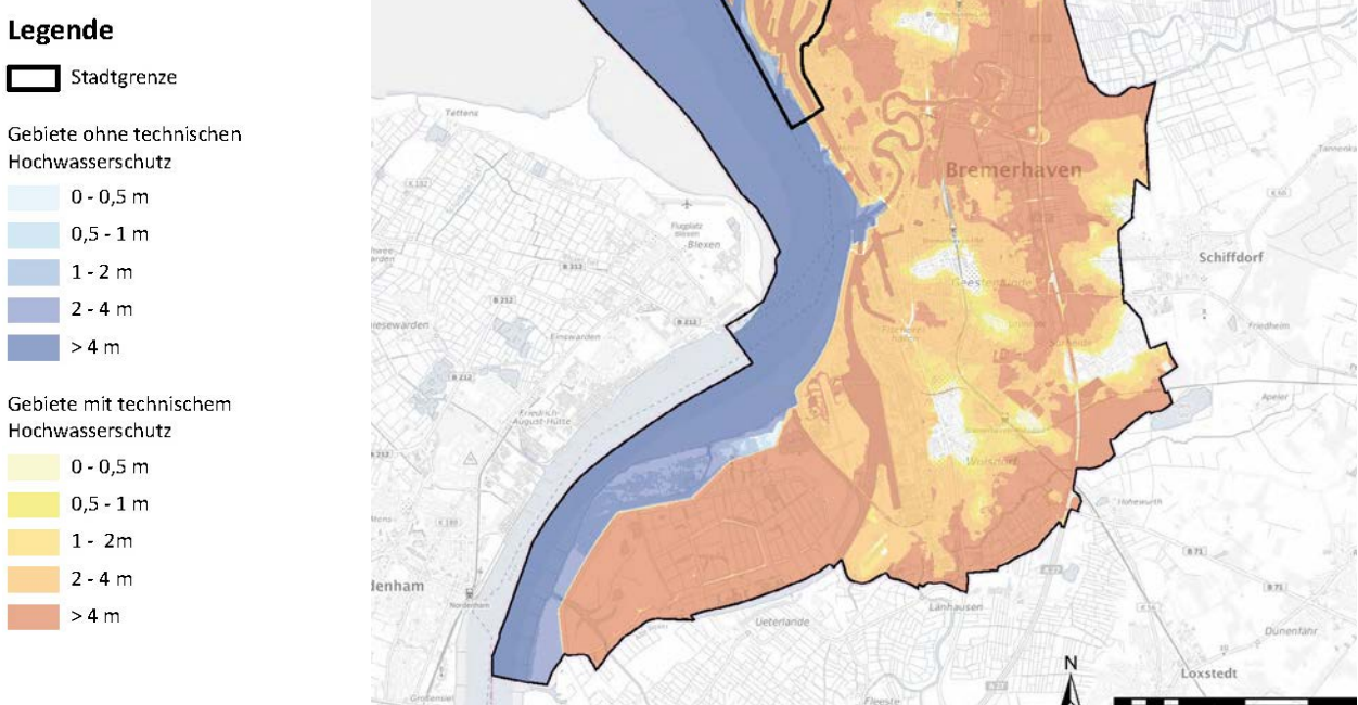
Abb. 41 Belastungskarte Flusshochwasser Bremerhaven
