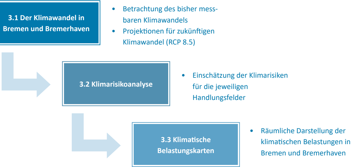
Abb. 19 Ebenen der klimatischen Betroffenheitsanalysen
