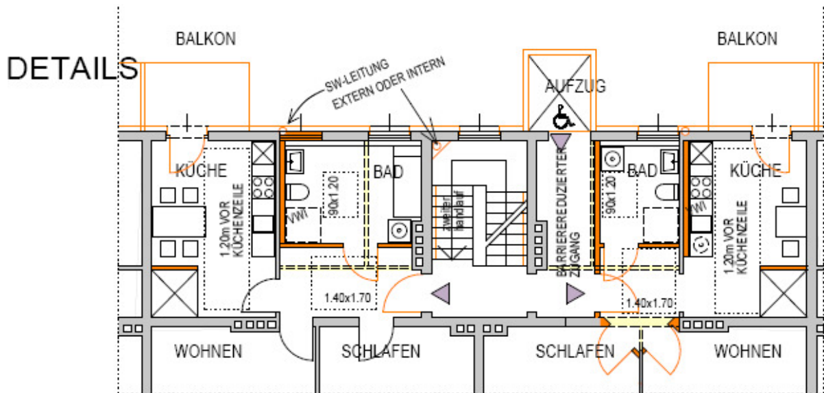
Grundrissdetail: Wohnung für Rollstuhlfahrer
