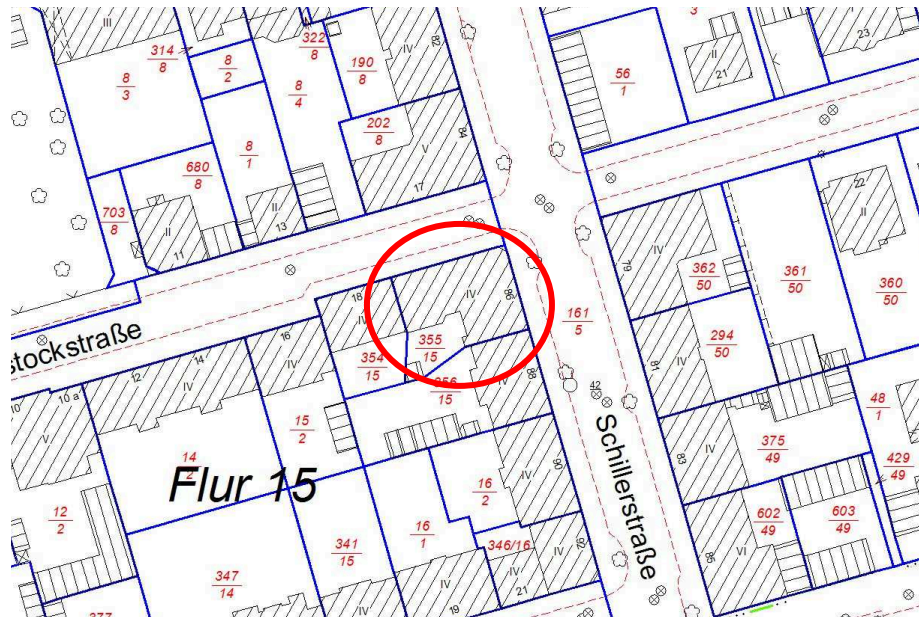
Lageplan Schillerstraße
