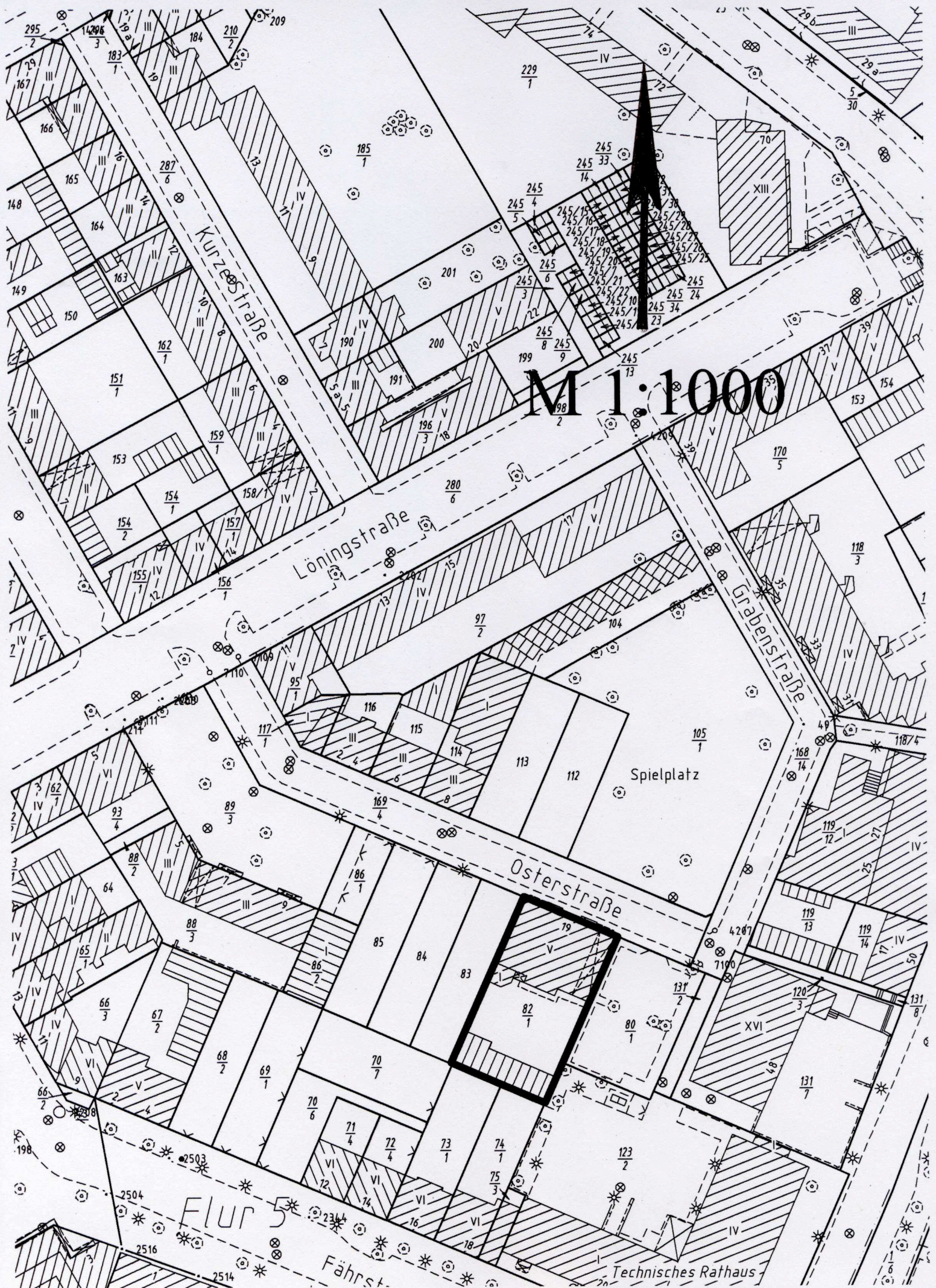
Anlage 4: Lageplan
