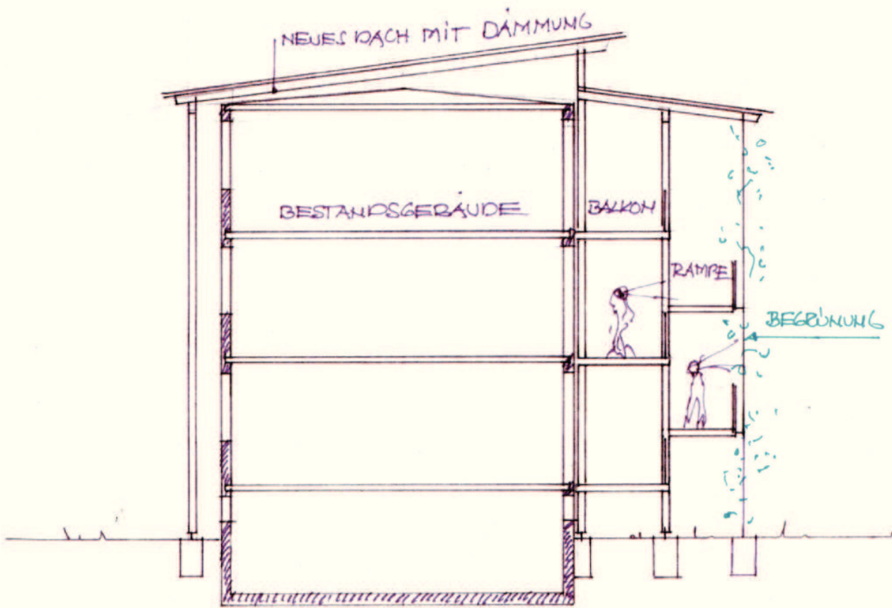
QUERSCHNITT RINGSTR. 36-40
