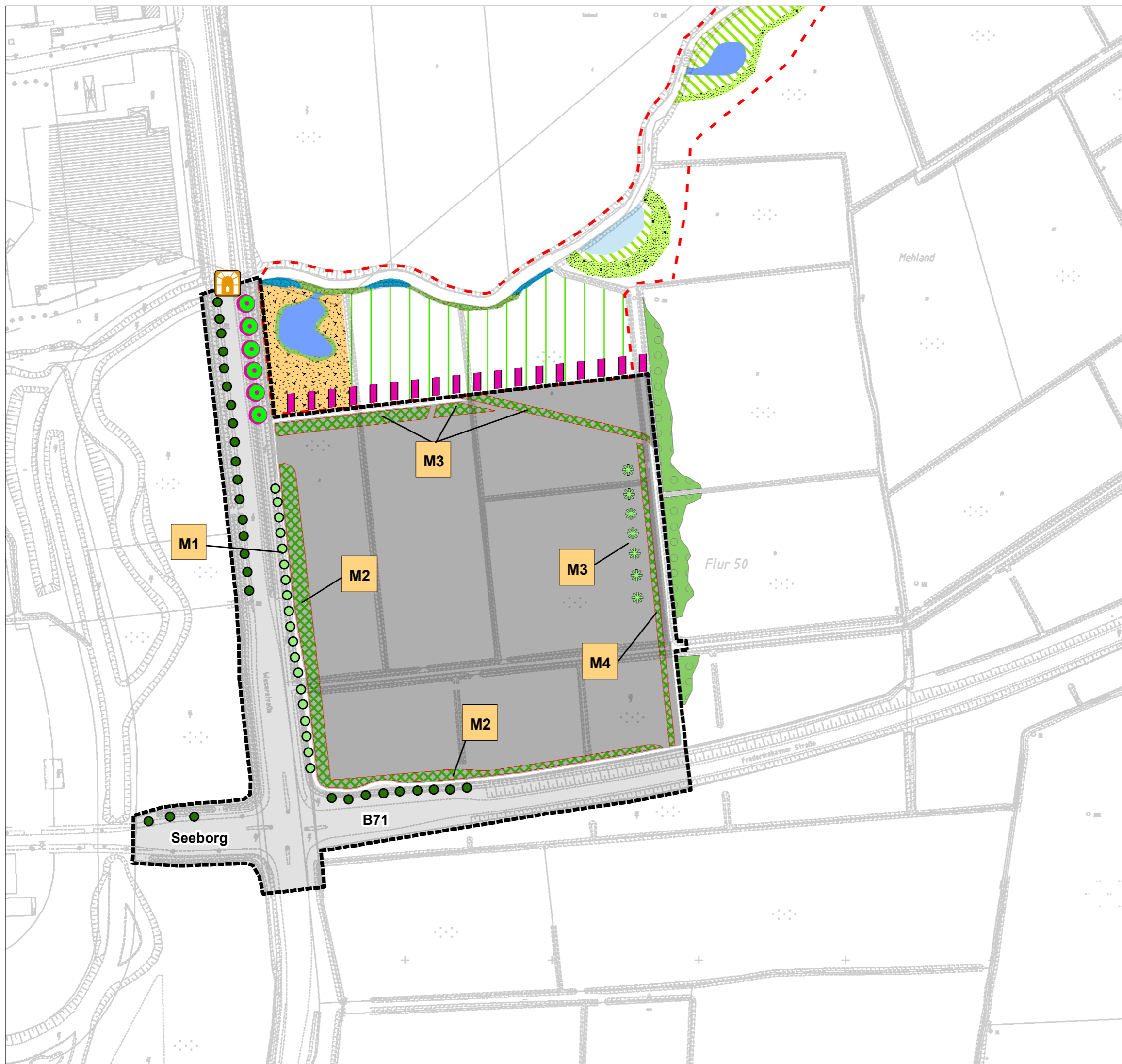
Abb. 8: Vermeidungs- und Kompensationsmaßnahmen im Geltungsbereich des B-Plans Nr. 444
